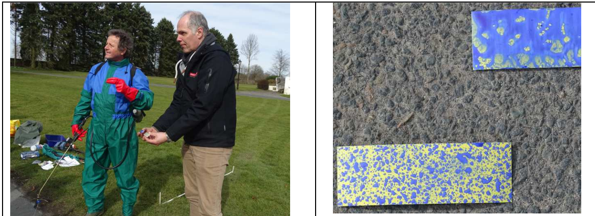
Abb.5: Spritzendruck und Laufgeschwindigkeit verändern das Spritzbild. Teststreifen unten optimal.
